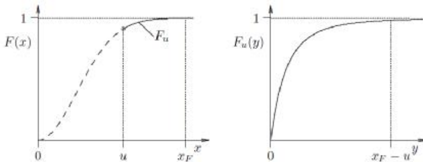
شکل (2): تابع توزیع احتمال F (سمت چپ) و تابع توزیع شرطی F_u (سمت راست)
