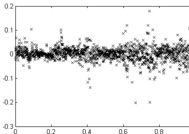
نمودار (1): چگالی اجزای اخلال با تخمین زننده رگرسیون کرنل
