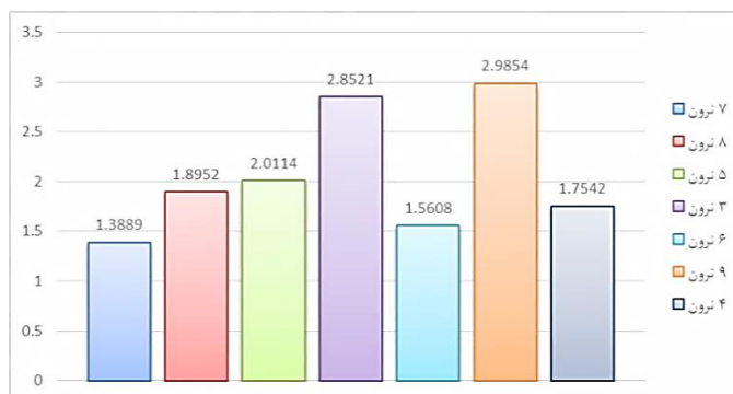
شکل ۱۰. مقایسه نتایج پیش‌بینی به‌دست‌آمده عامل شاخص قیمت در مدل دوم به ازای تعداد نرون مختلف
