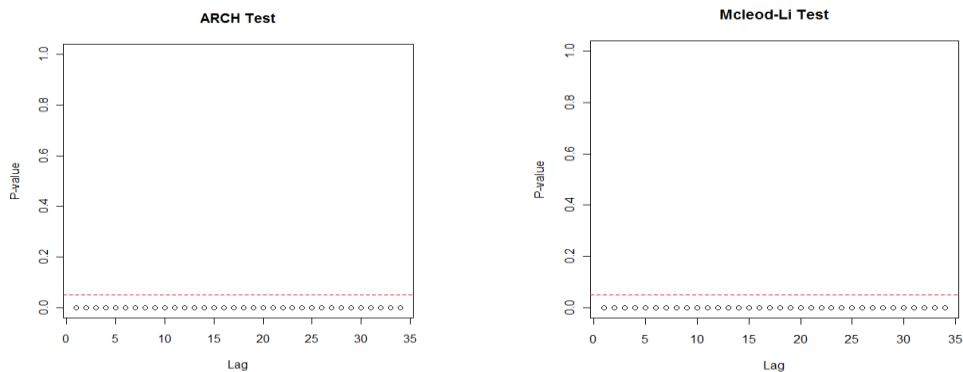
شکل (۴): نتایج آزمون اثر آرچ انگل در سری باقی مانده هانتایچ آزمون اثر آرچ مک لنود-لی در سری باقی مانده
