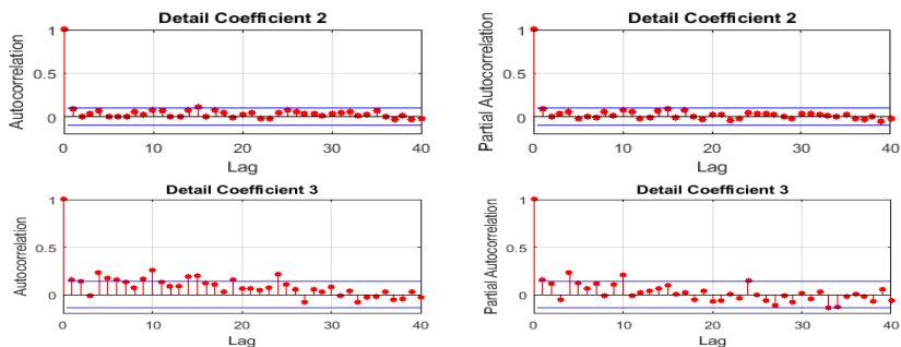
شکل (۷): شکل خودهمبستگی (چپ) و خودهمبستگی جزئی (راست) مربعات سری ضریب جزئیات مرحله
