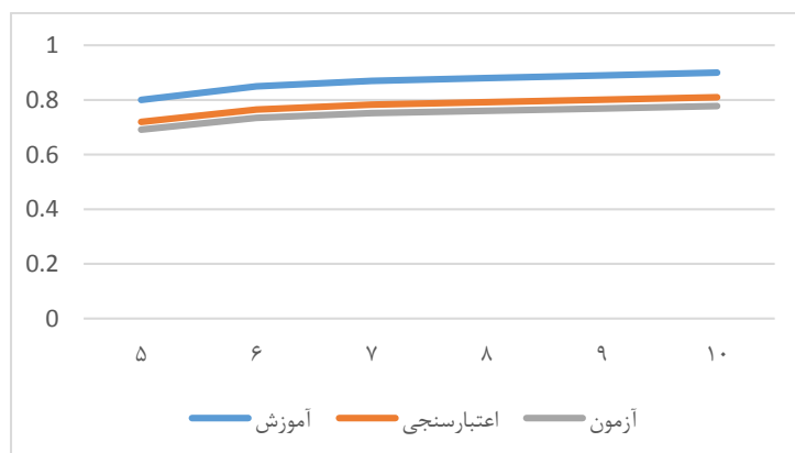
نمودار ۲. نتایج داده‌های آزمون، اعتبارسنجی و آموزش برای تعیین تعداد لایه‌های بهینه
