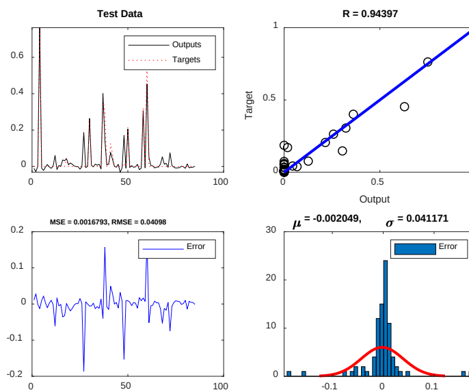
شکل ۱. نتایج اجرای الگوریتم عصبی با استفاده از روش لونبرگ
