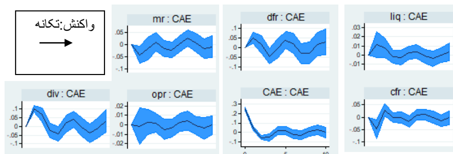
نمودار ۳. اثر تکانه متغیرهای پژوهش بر کارایی تخصیص سرمایه (با شاخص ناکارایی سرمایه گذاری) در سطح خطای ۵ درصد محاسبه شده در هر طرف با استفاده از شبیه سازی مونت کارلو با ۲۰۰ بار تکرار
