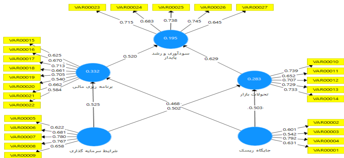
شکل ۲. تحلیل مدل در حالت ضرایب معناداری
